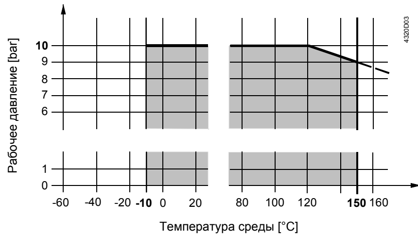
Рабочее давление для ISO 7005 при рабочих температурах -10 \dots +150 \text{ }^\circ\text{C} .
